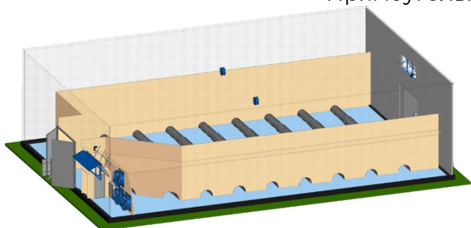
20x25, h-8 м поперечное расположение каналов
